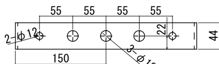
取付アーム部 孔ピッチ
