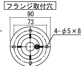
取付金具
