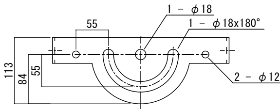
取付アーム部 孔ピッチ
